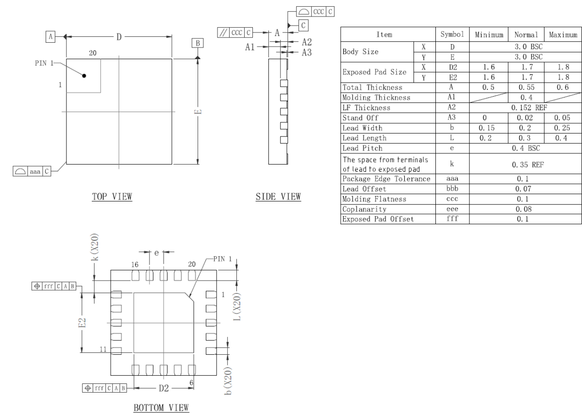
图 5-2: QFN20 封装图
